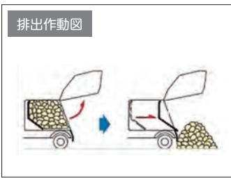
強制排出方式
