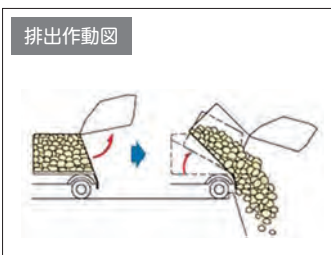
ダンプ排出方式
