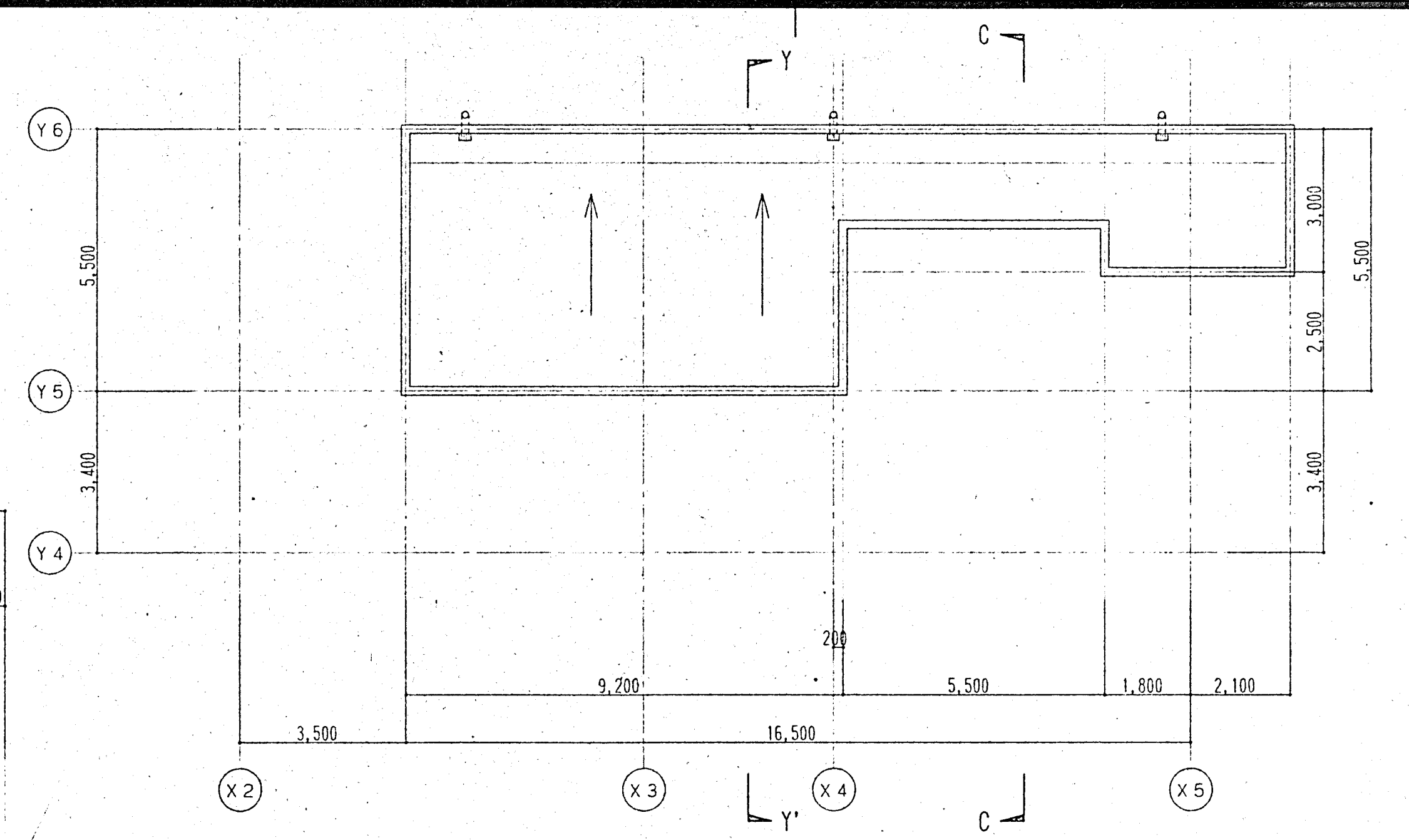
屋根平面図 S=1:100
