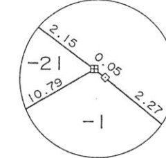
拡大図A
