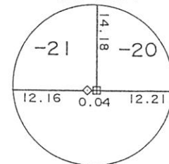
拡大図A
