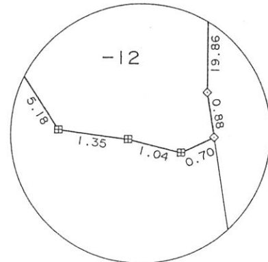
拡大図A
