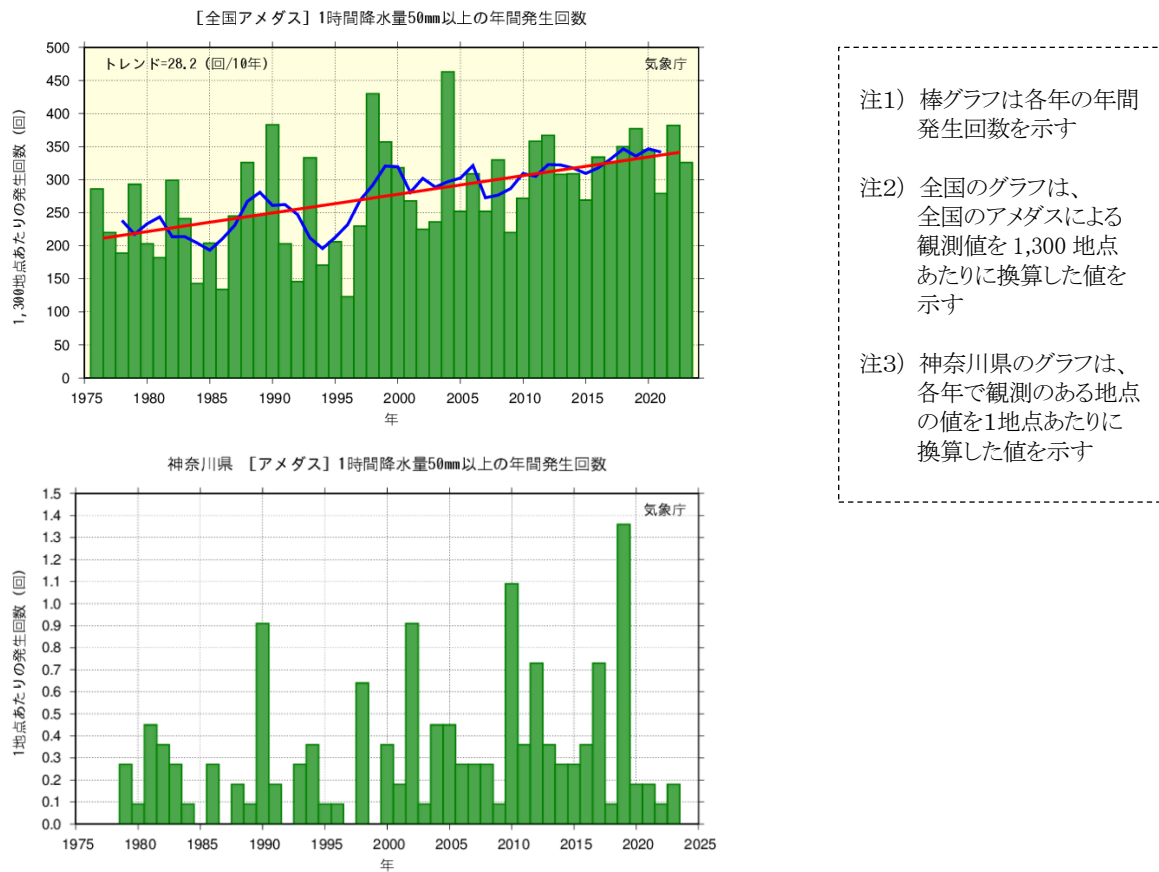
図2-16 【アメダス】1時間降水量 50 mm以上の年間発生回数 (上図:気象庁ホームページより 下図:東京管区気象台ホームページより)
