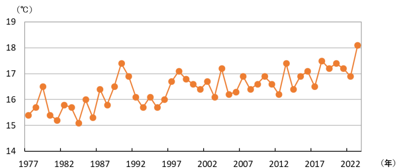
図2-17 横浜市の平均気温の変化
