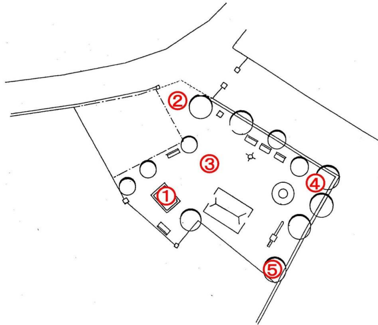
大津3丁目公園 平面図
