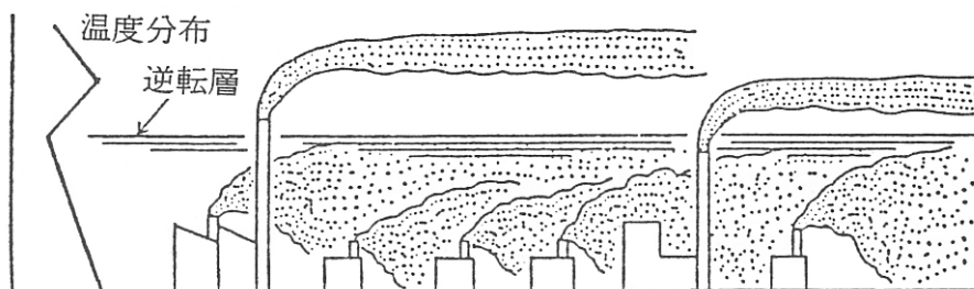
逆転層崩壊時のフュミゲーション
