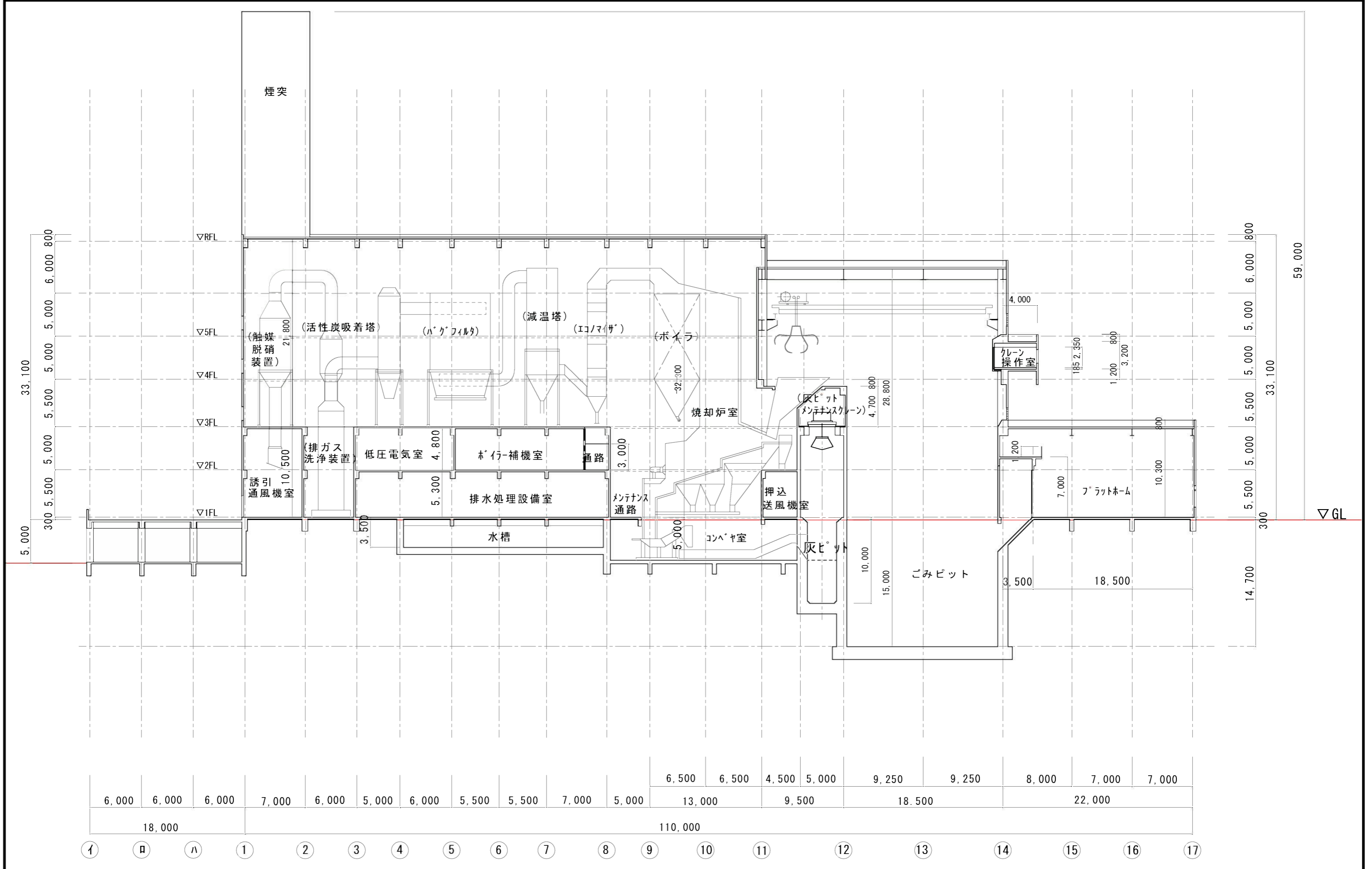
A-A 断面図 S=1/400
