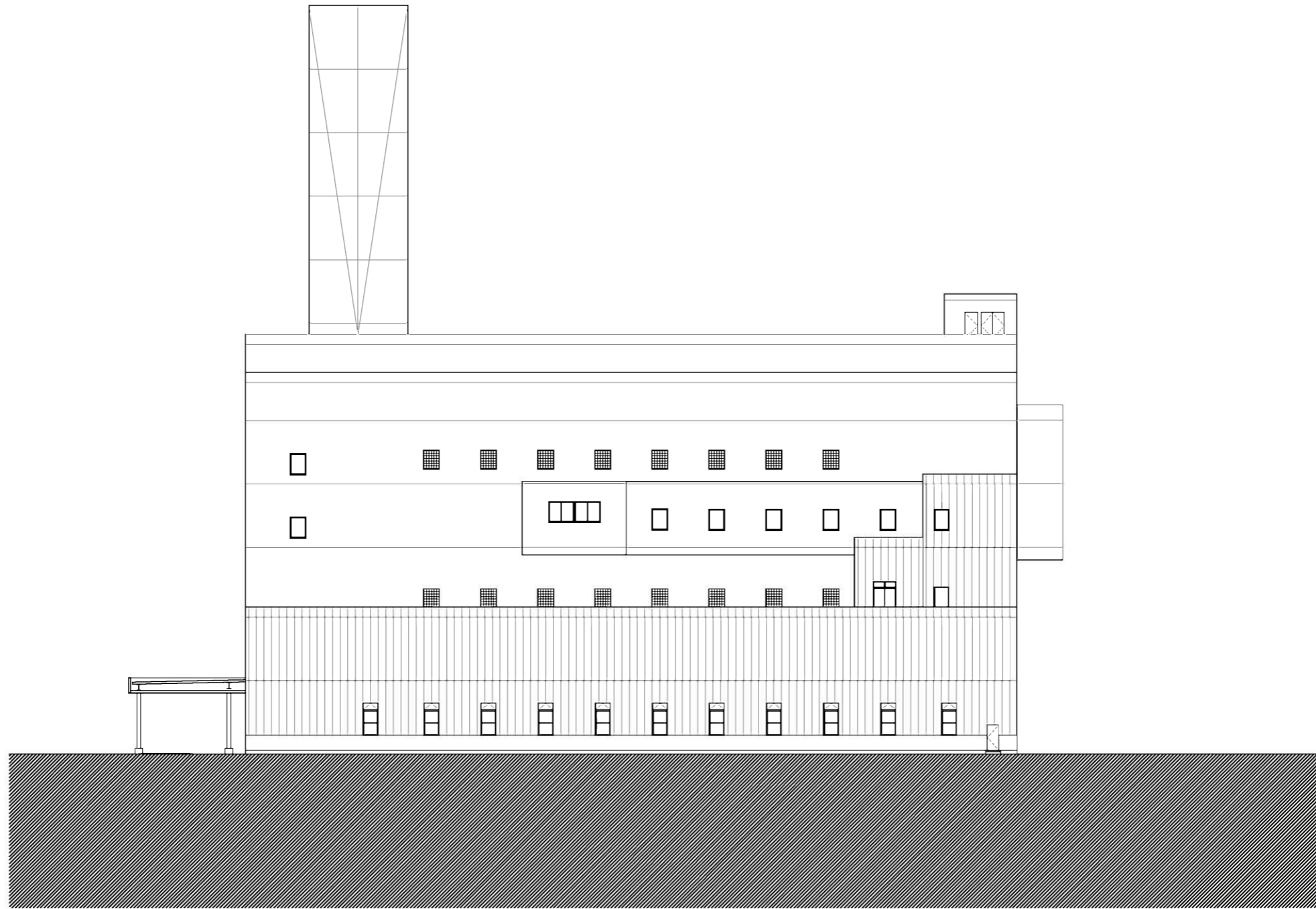
北立面図 S=1/400
