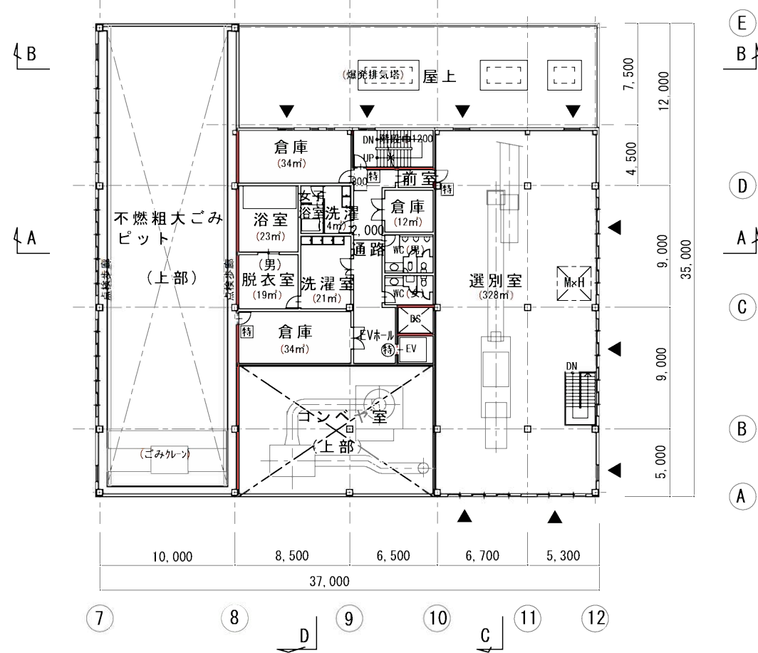
床面積 : 641.56㎡ 4階平面図 S=1/400
