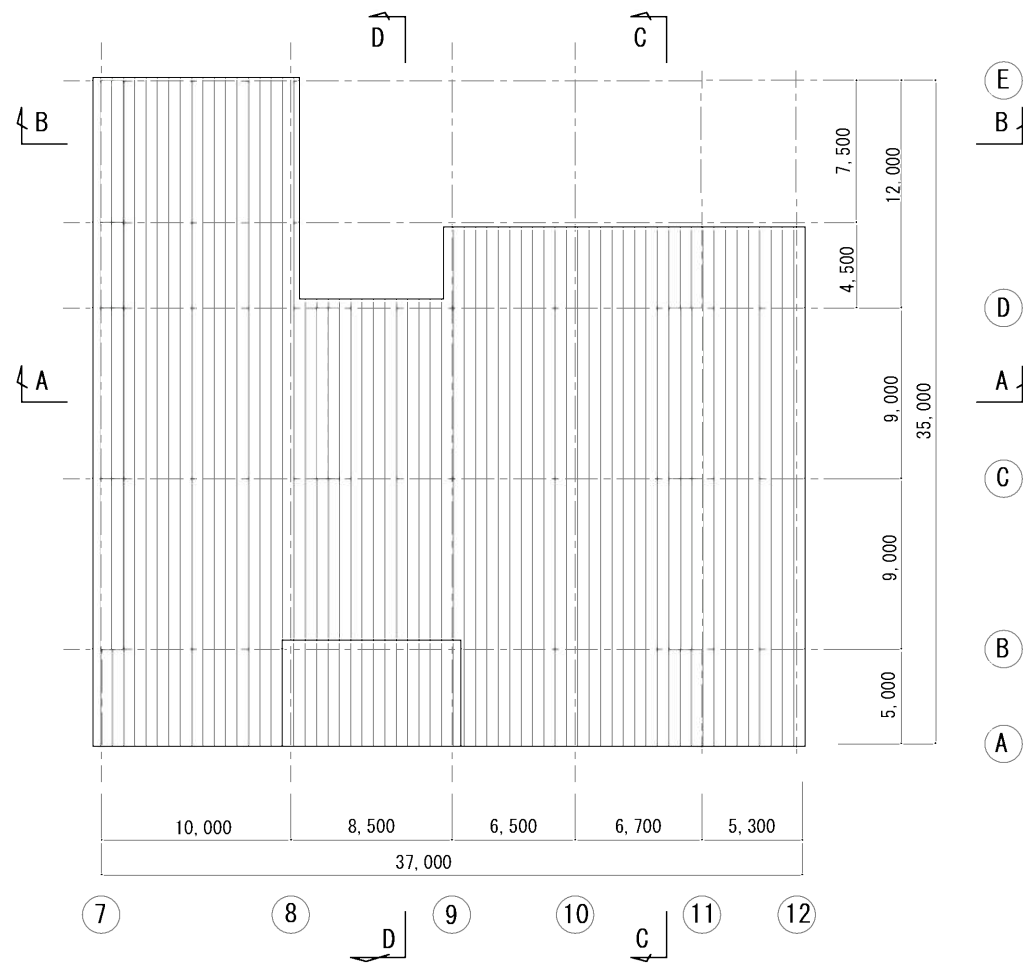
R階平面図 S=1/400
