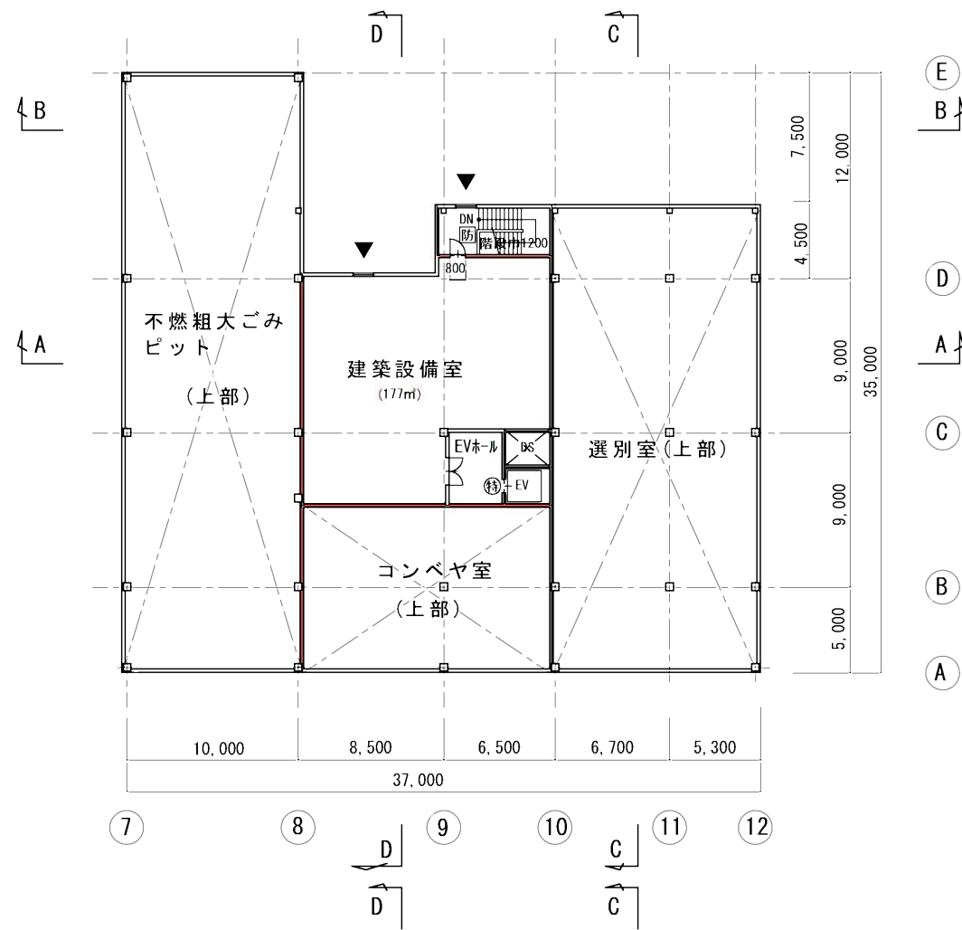
床面積 : 223.17㎡ 5階平面図 S=1/400
