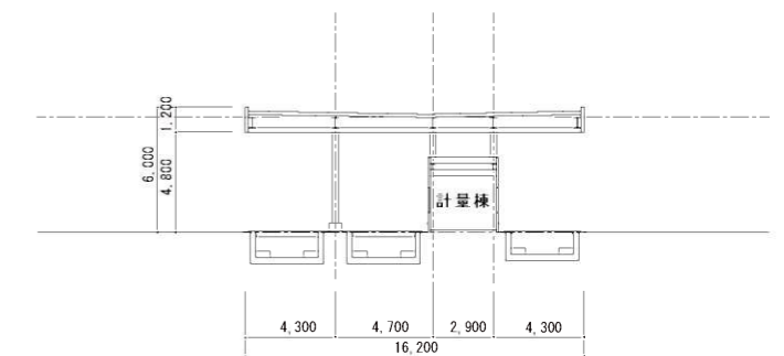
X-X 断面図 S=1/400
