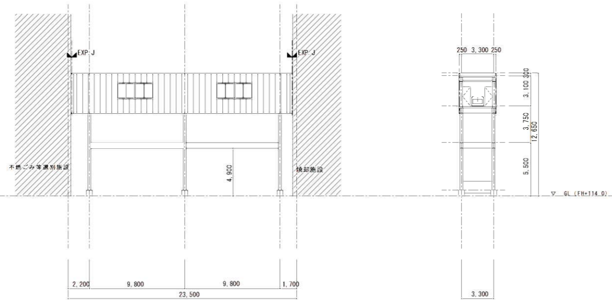
連絡橋 立面図 S=1/400
