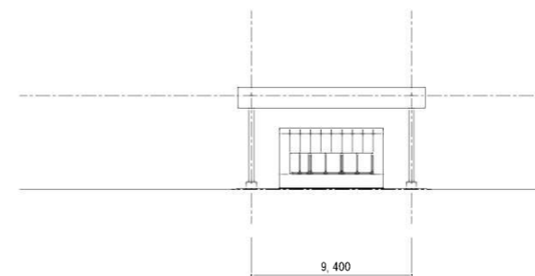
立面図 S=1/400
