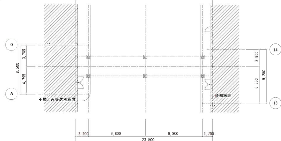
連絡橋 平面図 (FH+114.0)
