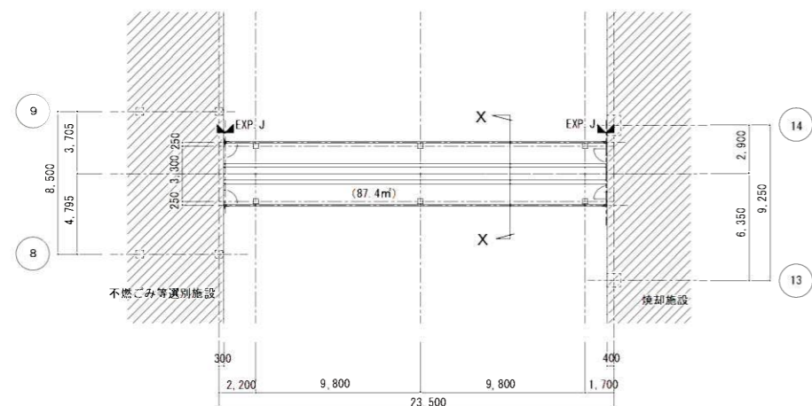
連絡橋 平面図 (FH+124.0)
