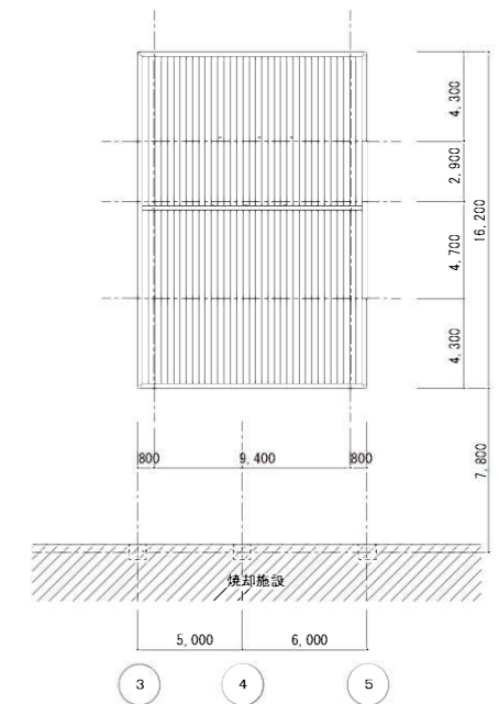
屋根伏図 S=1/400
