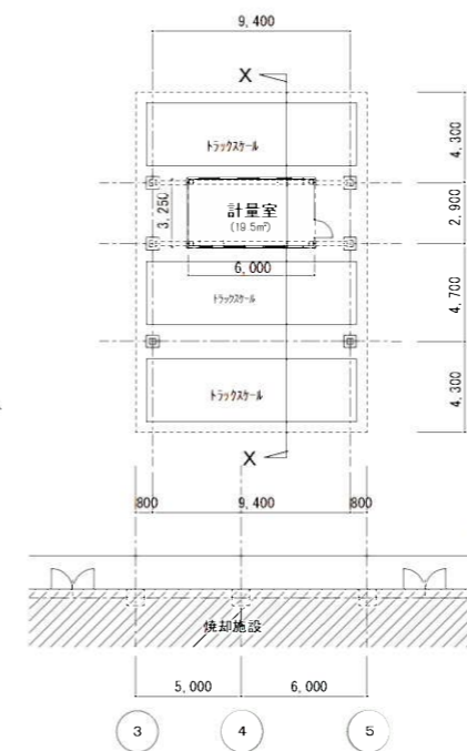
平面図 S=1/400
