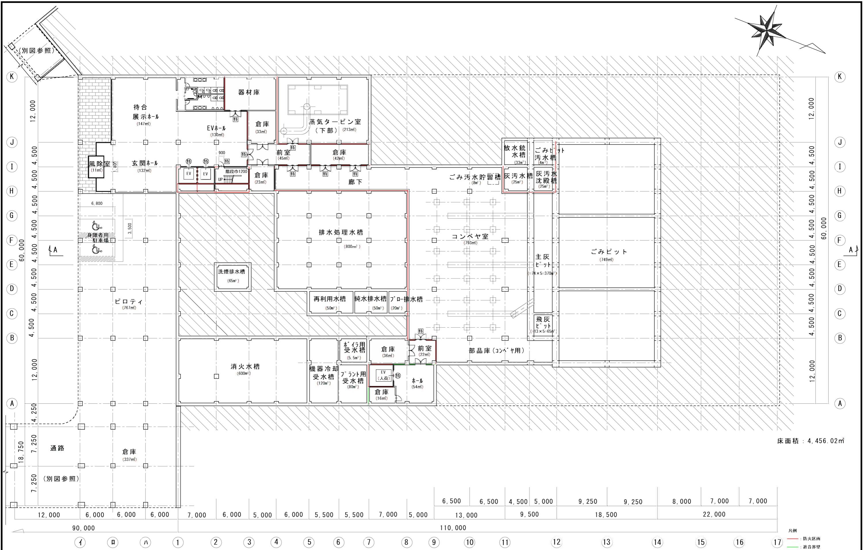
地下1階平面図 S=1/400
