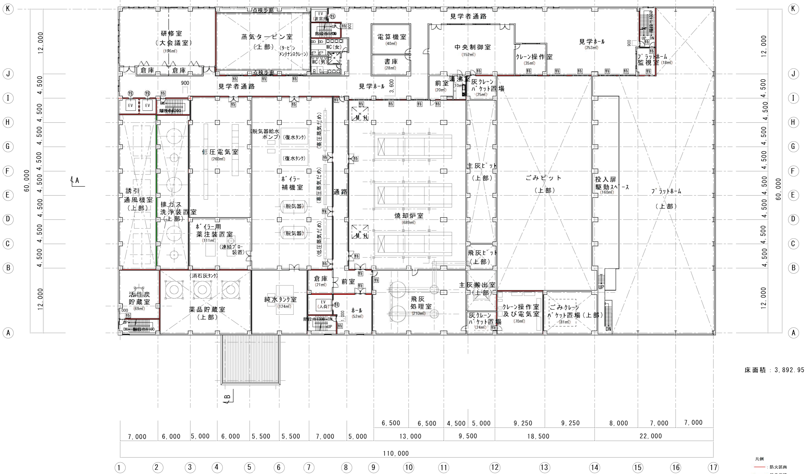
2階平面図 S=1/400
