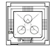
煙突基準平面図 S=1/400
