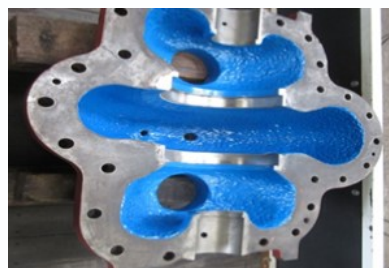
FC製ポンプケーシング 補修後
