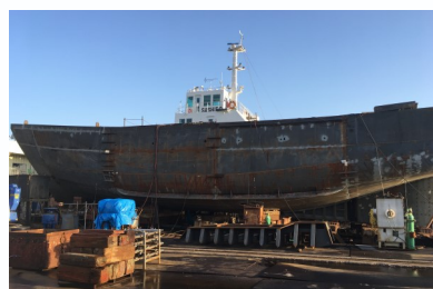
船殻製造の様子
