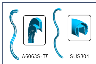
異形断面の3次元形状加工
