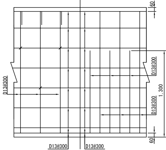
たて壁配筋図 前面 背面
