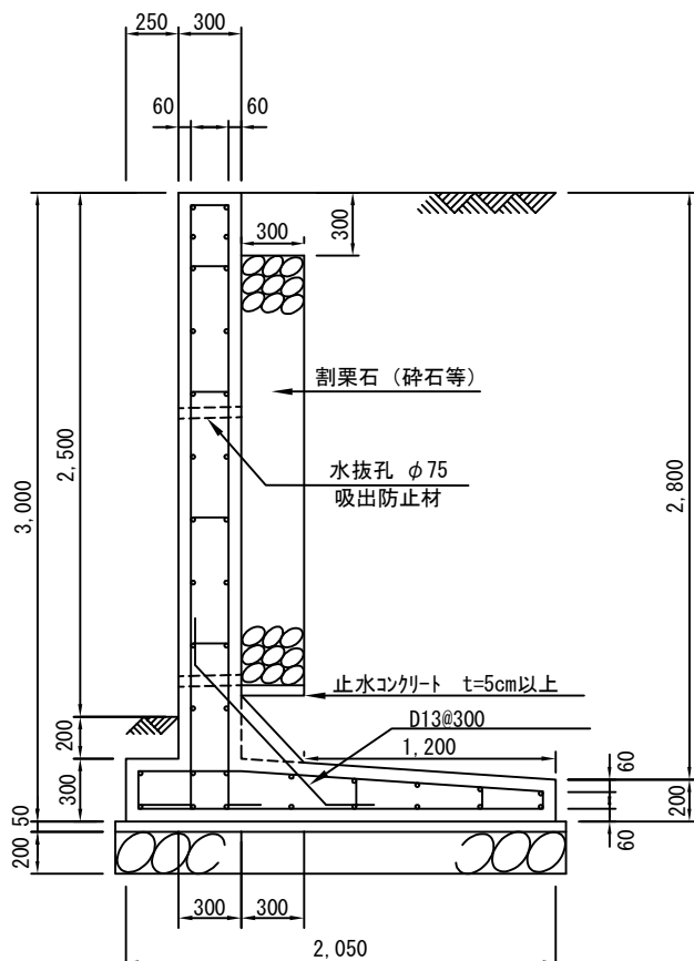
底版配筋図
