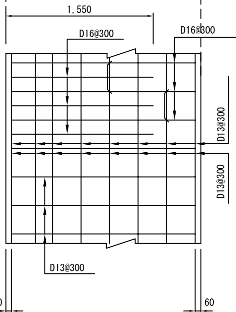
底版配筋図
