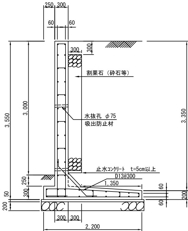
底板配筋図
