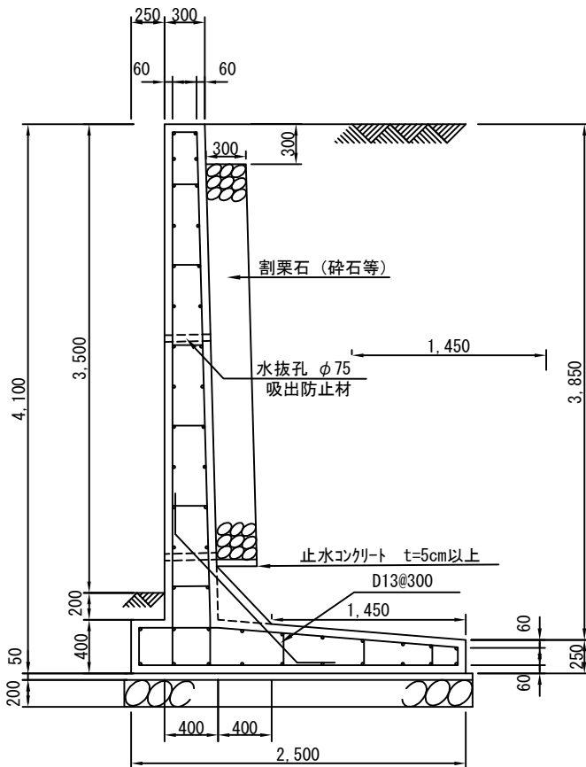
底板配筋図
