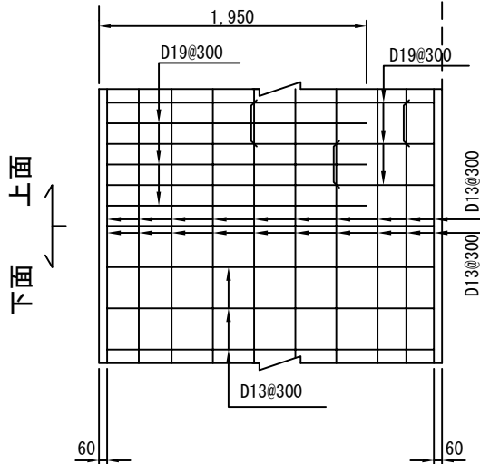
底板配筋図
