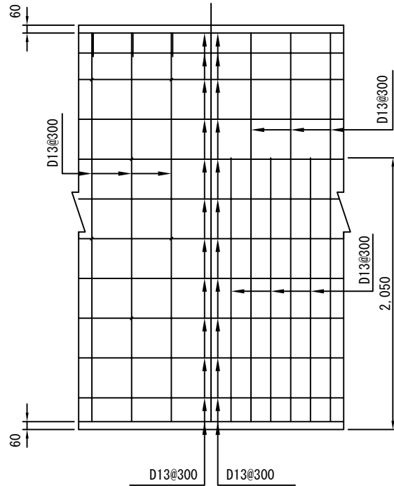
たて壁配筋図 前面 背面
