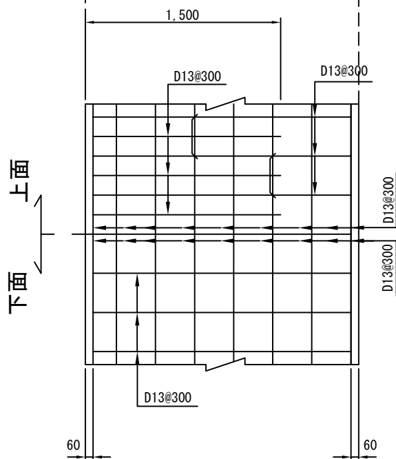
底板配筋図
