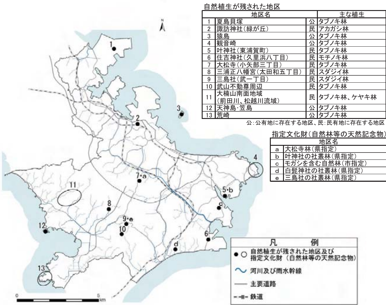
自然植生が残された地区及び自然林等の天然記念物
