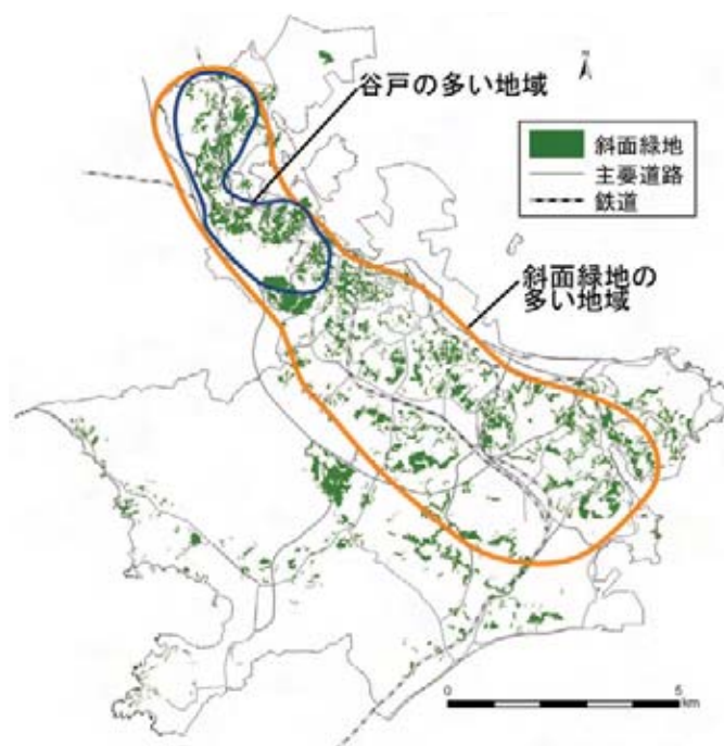
斜面緑地と谷戸地域の現況
