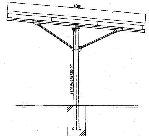
側面図
