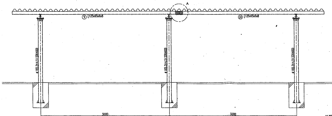
正面図
