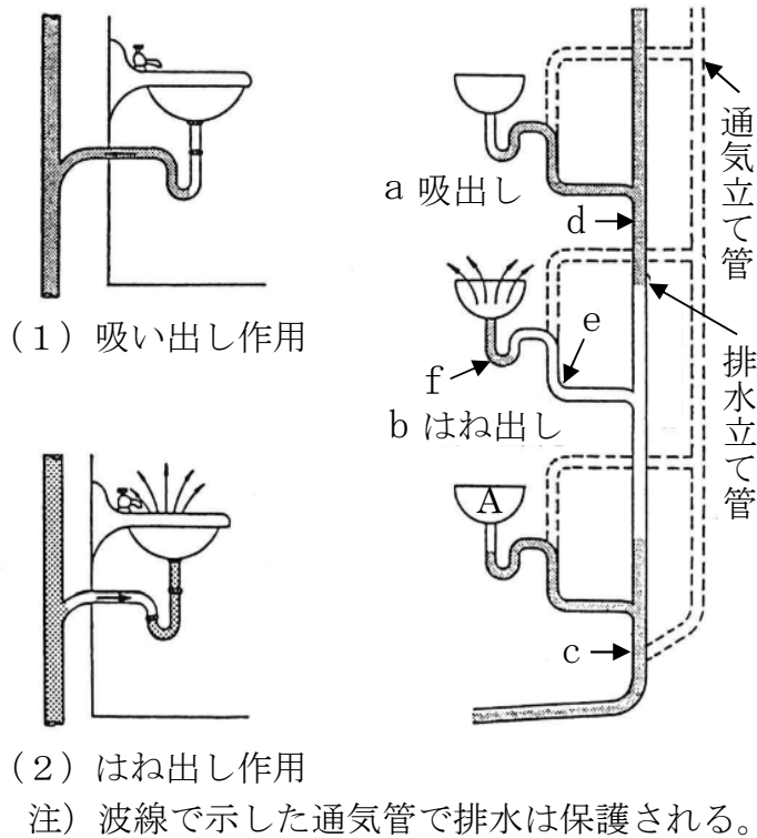
図3-5 はね出し作用と吸い出し作用
