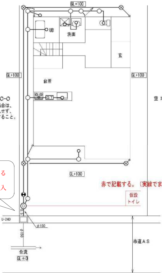
1 F 平面図
