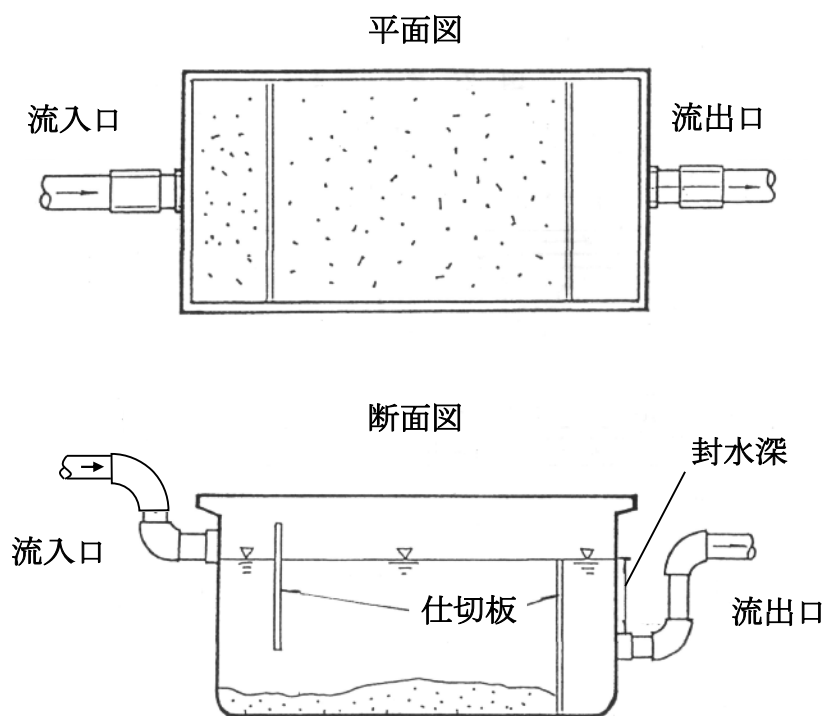
図 3-26 砂阻集器
