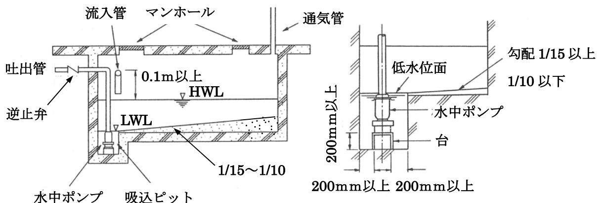
図3-30 排水槽の例
