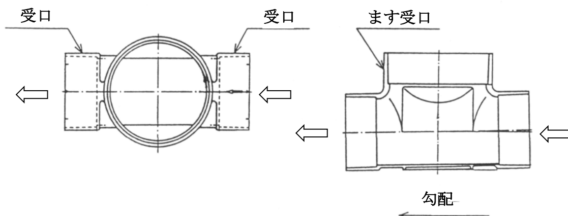
図3-36 中間ます
