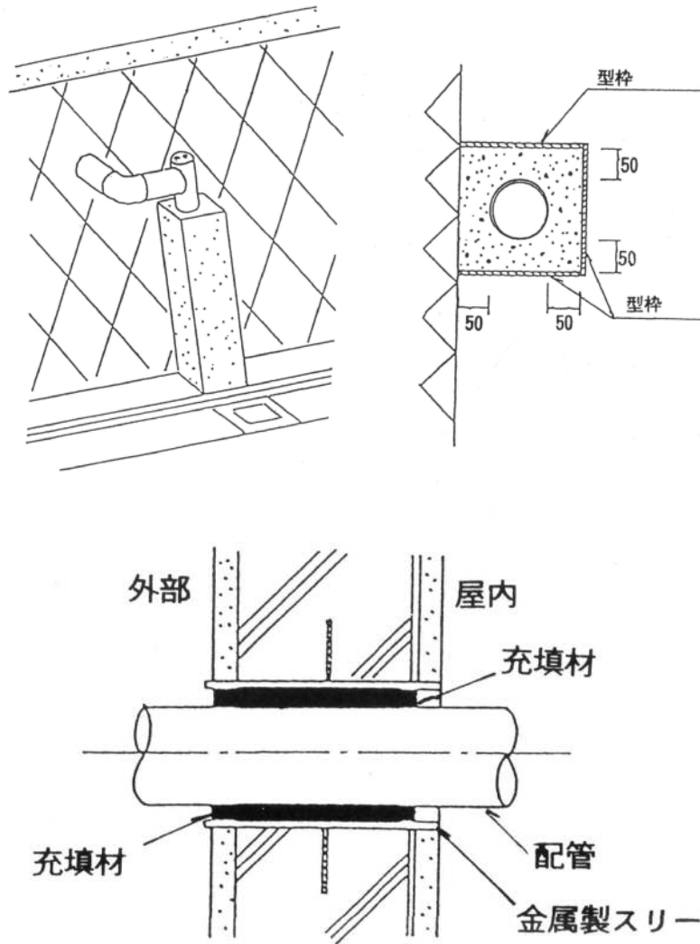
図4－6 防護工
