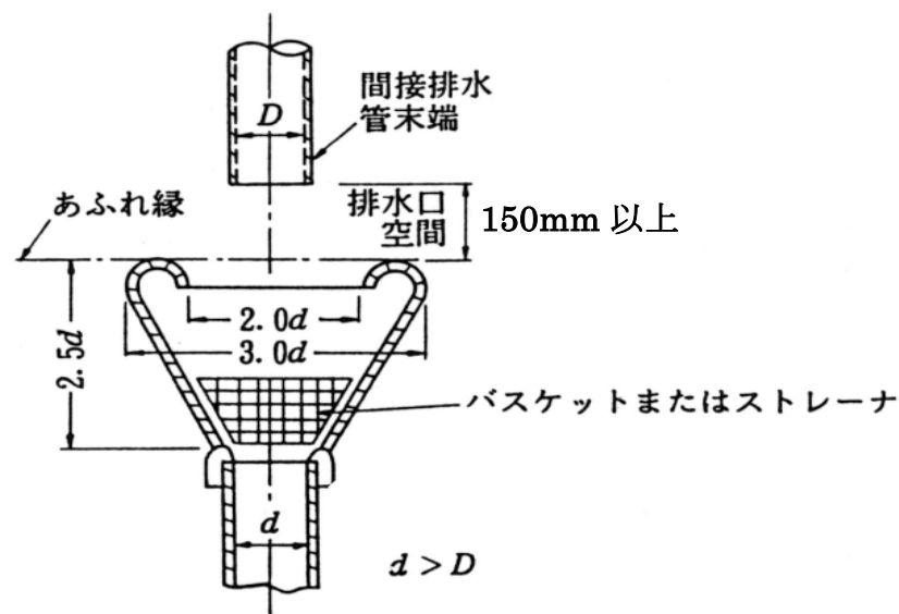
図 3－32 排水口空間
