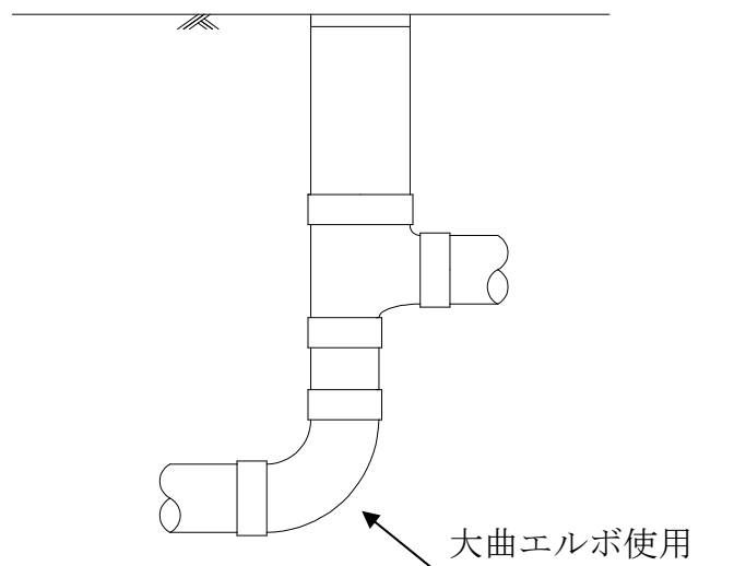
図 3 - 42 ドロップマス設置例
