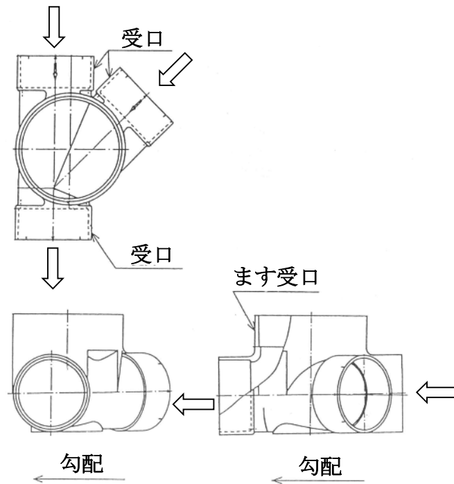
図3-37 合流ます
