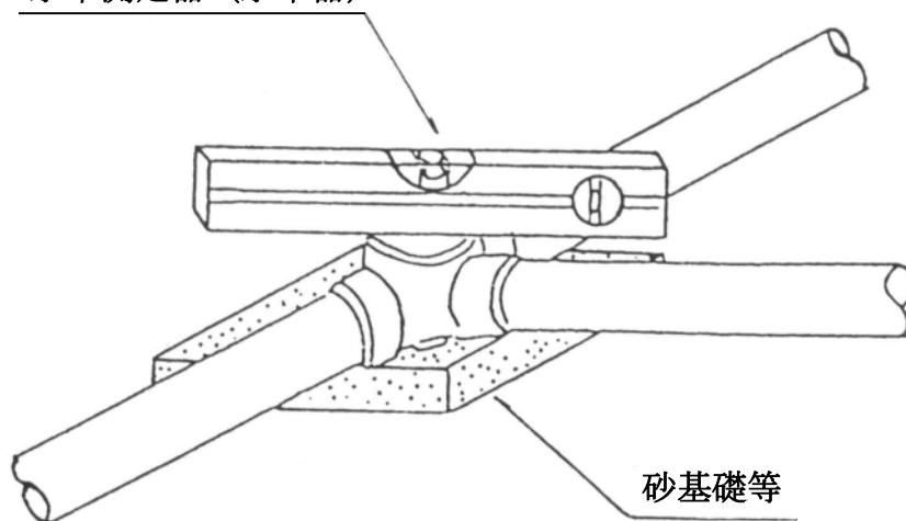
図4-7 基礎工
