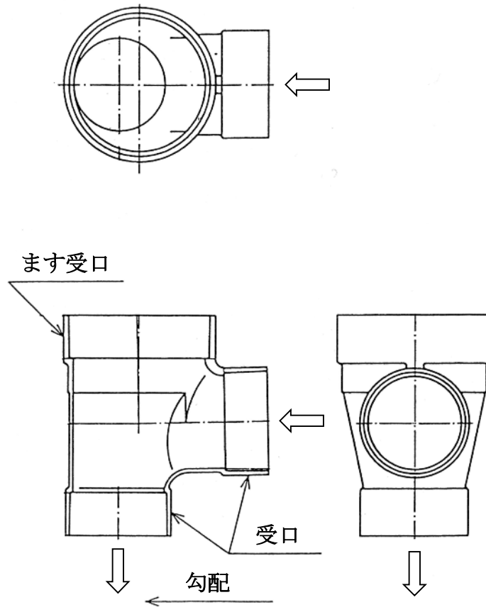
図 3 - 41 ドロップマス
