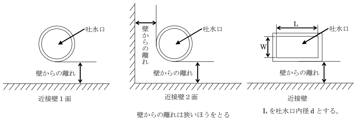
図 8・8・1 吐水口空間
