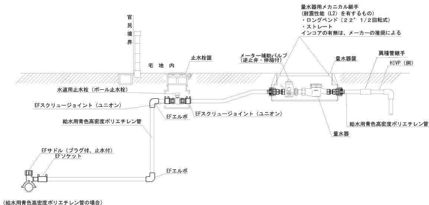
図1 配水管分岐からの標準図
