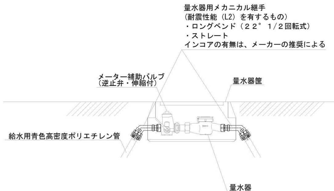
図2 量水器廻り標準図
