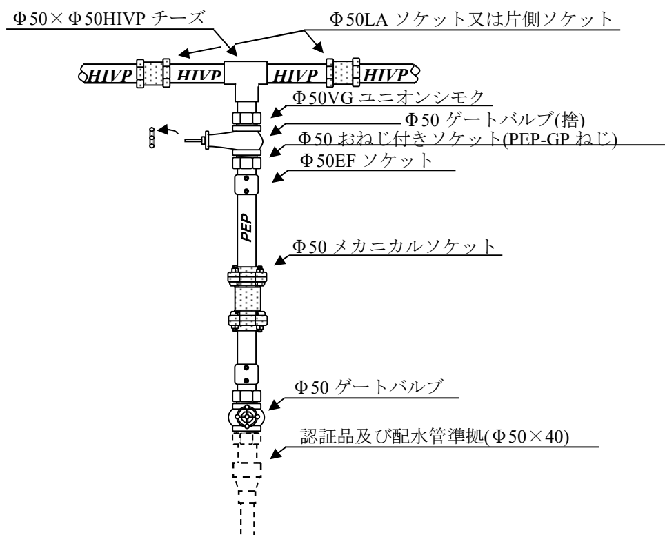
図 12・4・2 道路横断部 HIVP 切断分岐 (PEP 使用時)
