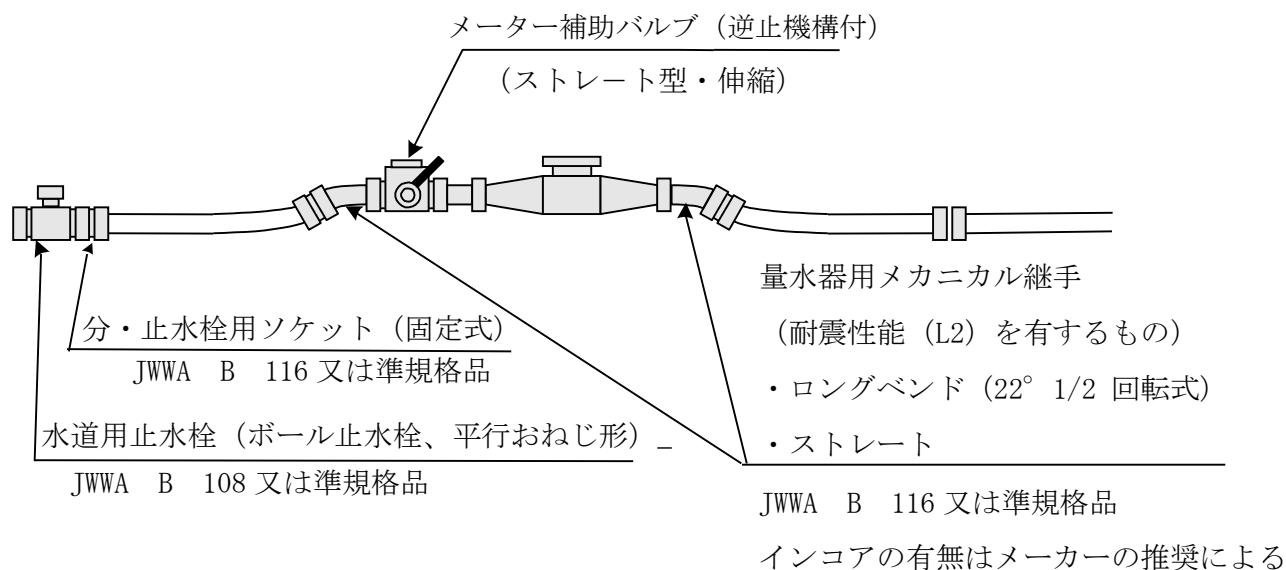
図 11・5・2 止水栓、水道メーター間の配管
