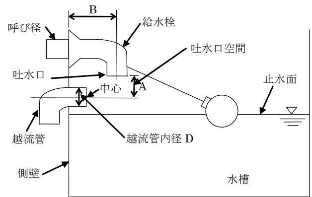
(3) 水槽の場合（越流管横取出し）
