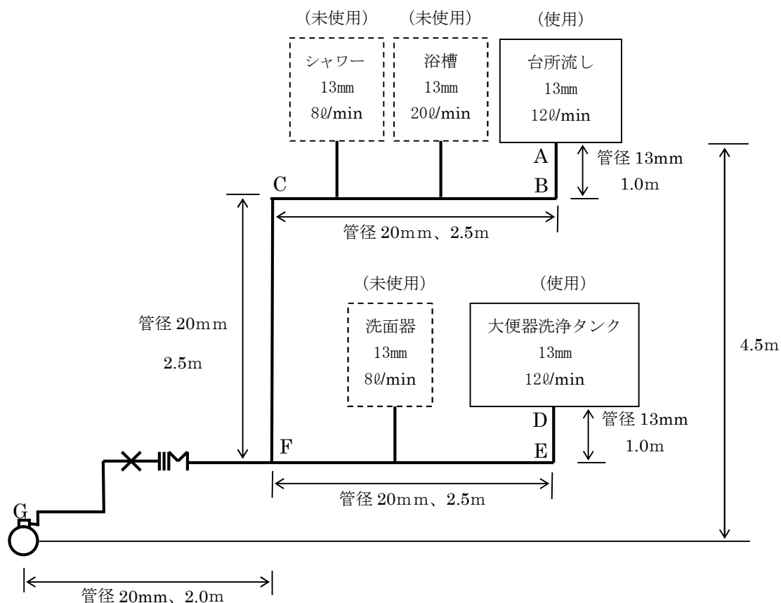
図 3・4・4 給水装置概要図
