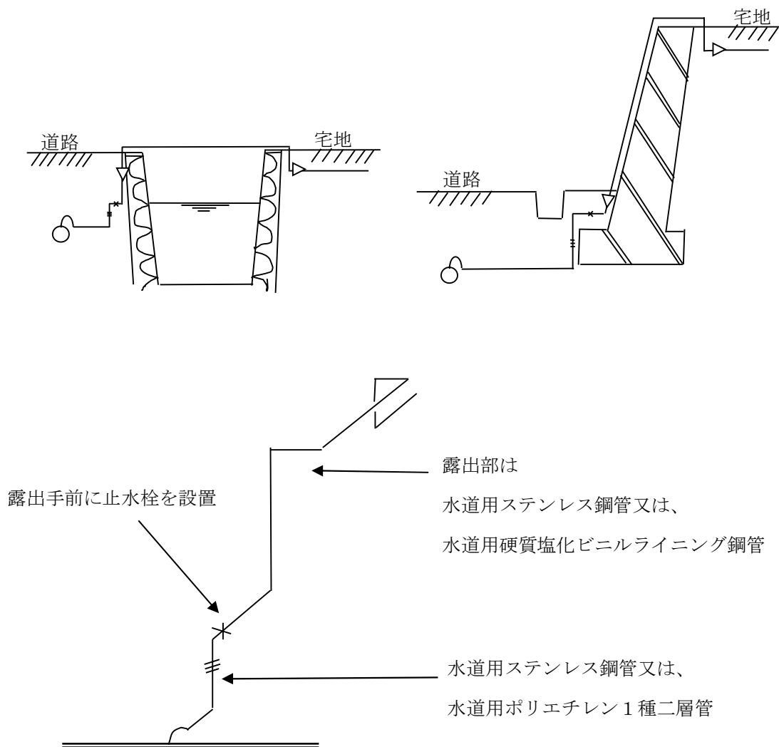
図 8 ・ 5 ・ 6 河川、石垣等の配管例
