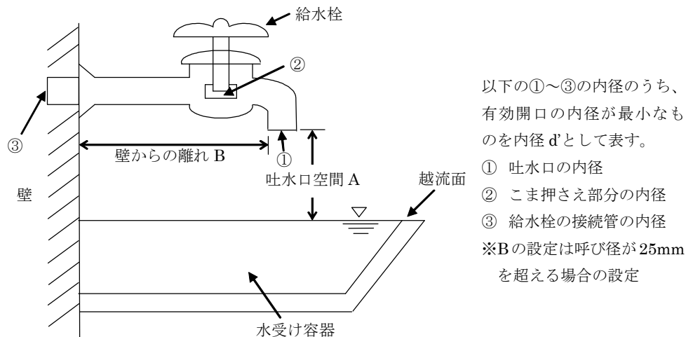
(1) 洗面器等の場合
