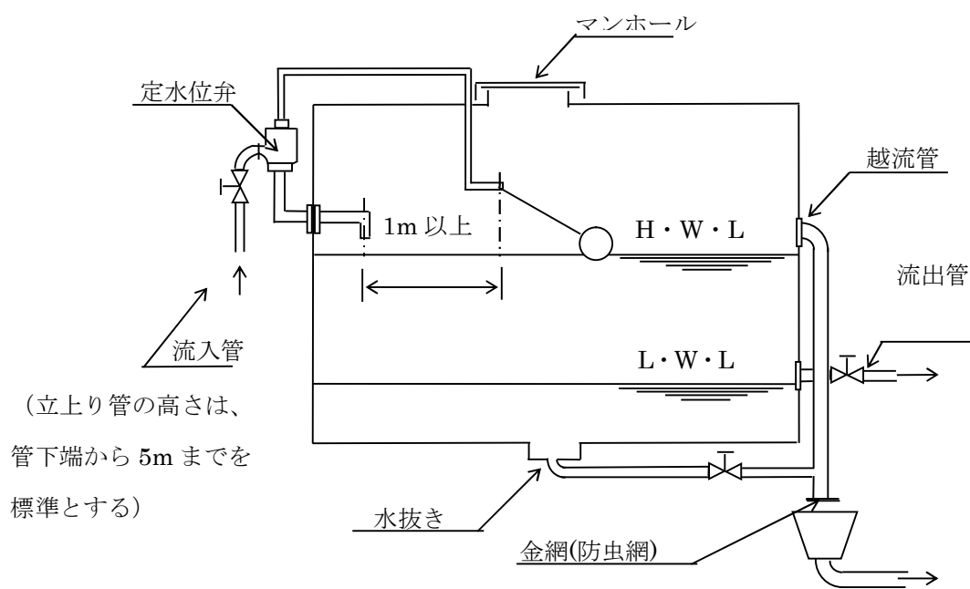
図 6 ・ 4 ・ 2 受水槽構造参考図（２）
