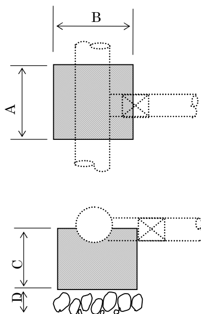
図 8・5・4 不断水割 T 字管防護標準図
