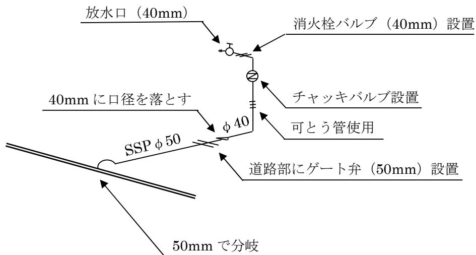
図 8・10・1 私設消火栓の構造
