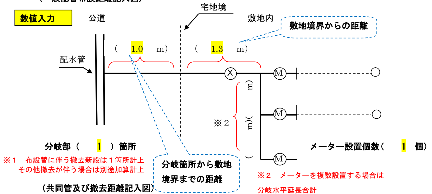
(一般配管布設距離記入図)
