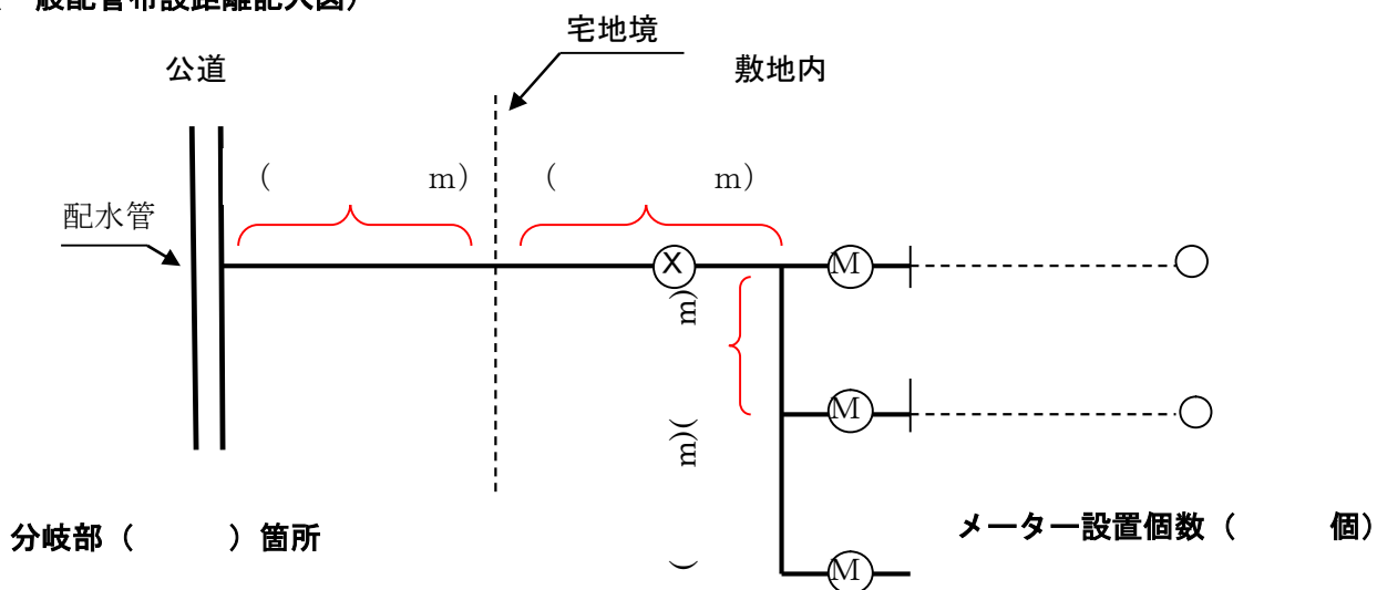
(一般配管布設距離記入図)
