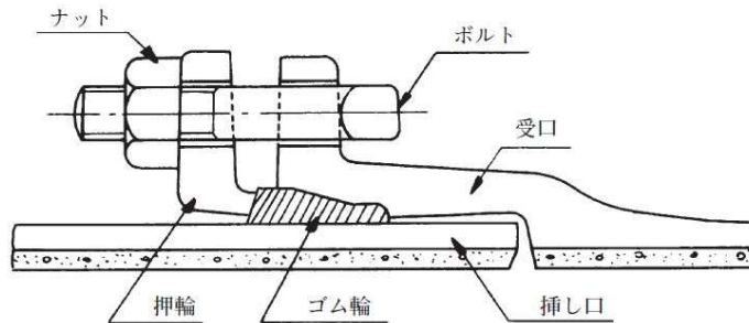
図1-1-1 継手の構造
