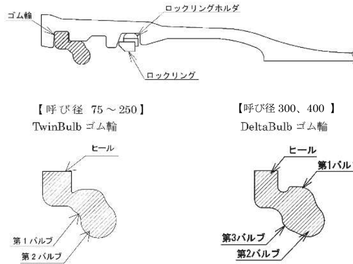
図1-2-4 ゴム輪のセット
