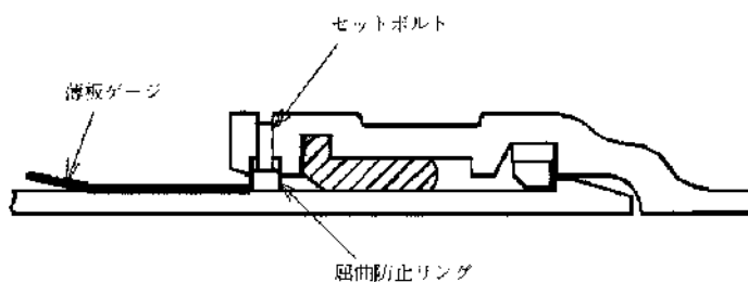
図 1-3-11 セットボルト締め付け確認（直管挿し口の場合）
