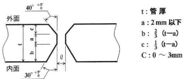
図3-1-1 開先標準図
