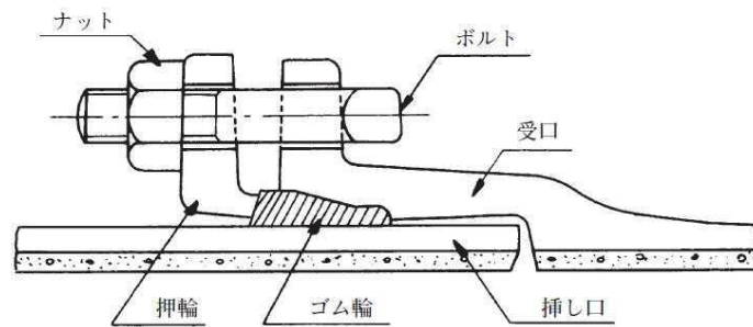
図1-1-1 継手の構造
