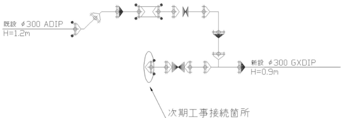
図4-5 次期工事用分岐配管例
