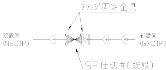
図４－７ （参考）既設耐震管接続部へのフランジ固定金具設置例
