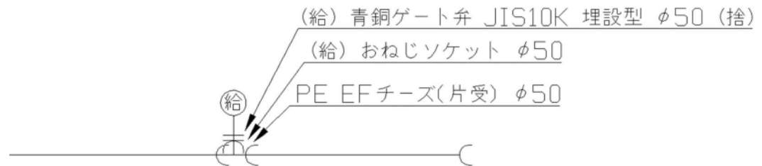
図4-1 (参考) \phi 50 の給水管への分岐配管図
