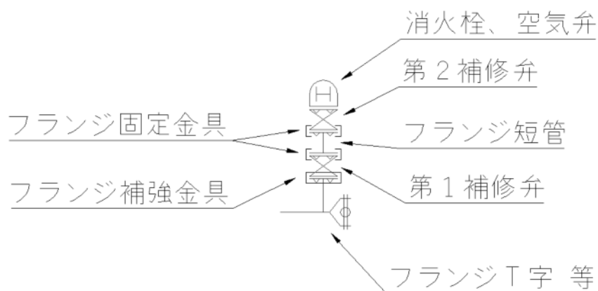
図４－８ （参考）消火栓・空気弁設置例
