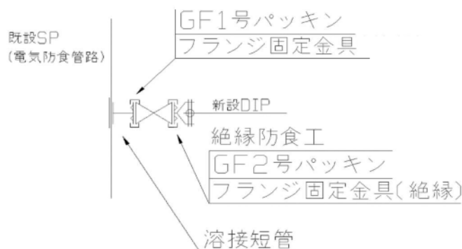
図4-6 （参考）電気防食管路からの分岐部における絶縁の例
