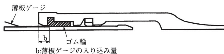
図 1-3-7 ゴム輪の位置確認
