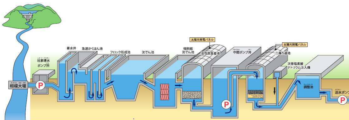
有馬浄水場の浄水処理
