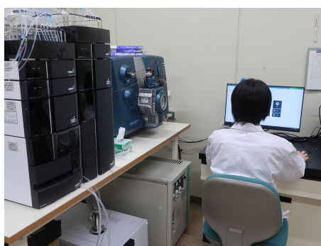
高速液体クロマトグラフ質量分析装置 （消毒副生成物、農薬の検査）
