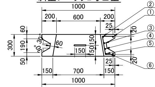
斜型ブロック2号乙型
