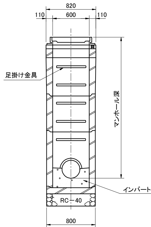
縦断面図
