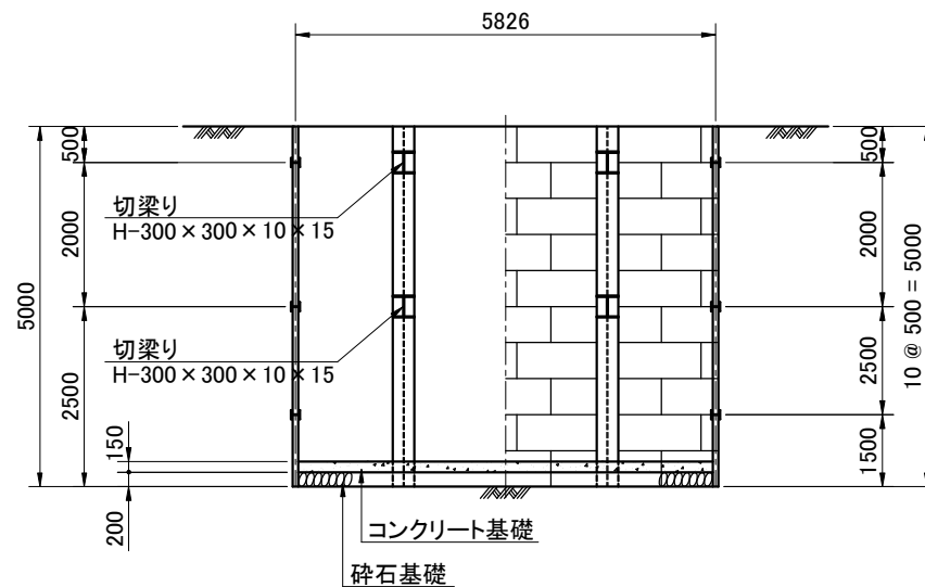
1 - 1 断面図
