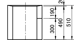
継手ブロック角1-2号 (360×460×510)
