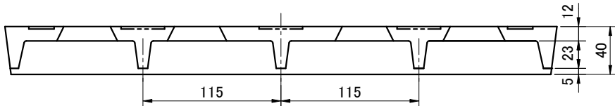
断面
