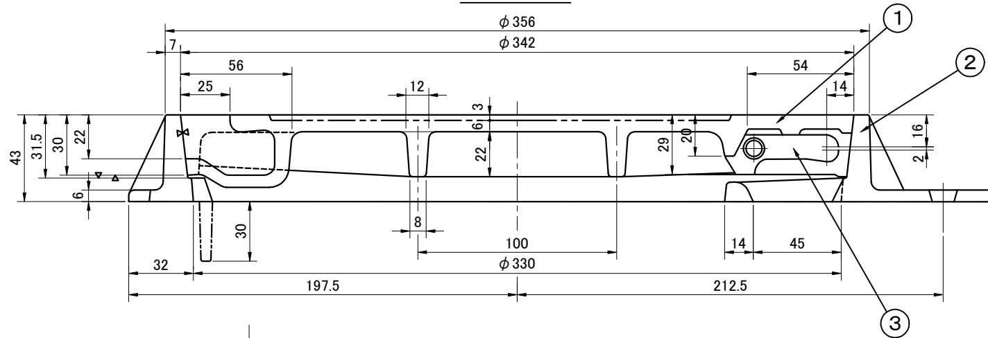
固定穴詳細
