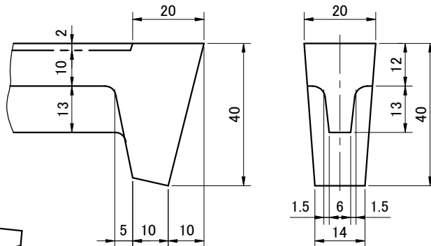
脚部詳細
