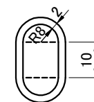
固定穴詳細
