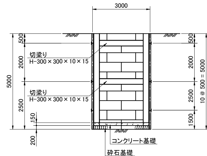
2 - 2 断面図
