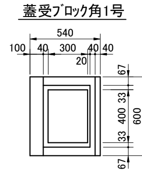
角 1 号 (L 型側溝コンクリート巾40cm)
