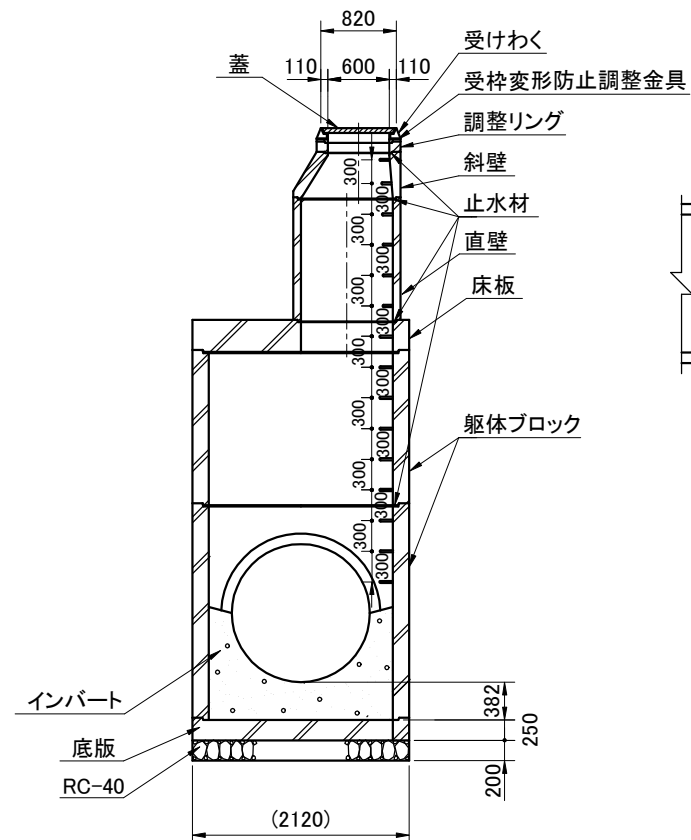
横断面図
