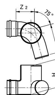
差し口形
