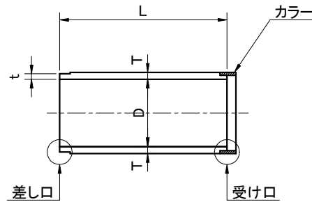
小口径管
