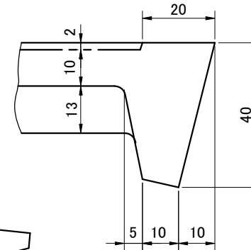
脚部詳細
