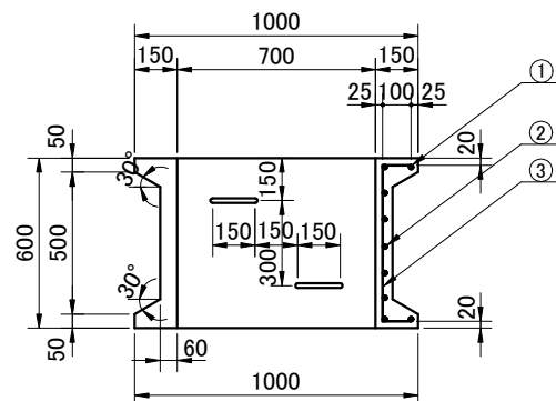
1号甲型
