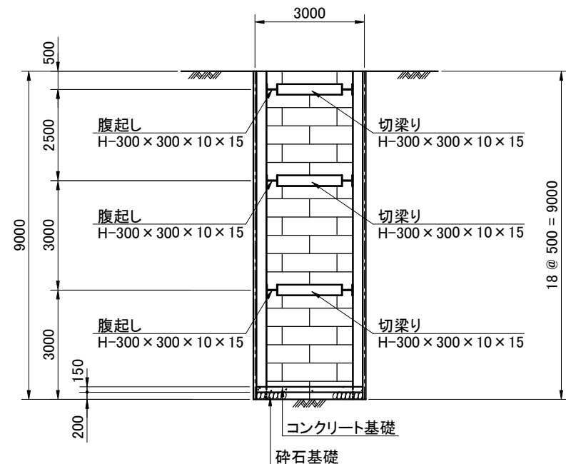
2-2 断面図
