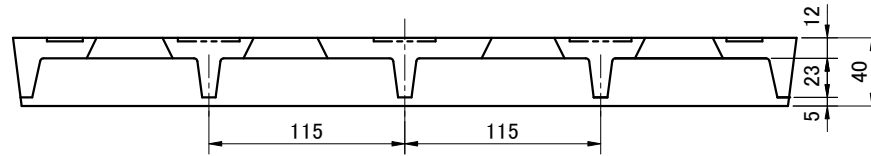
断面
