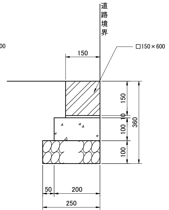
丙 型
