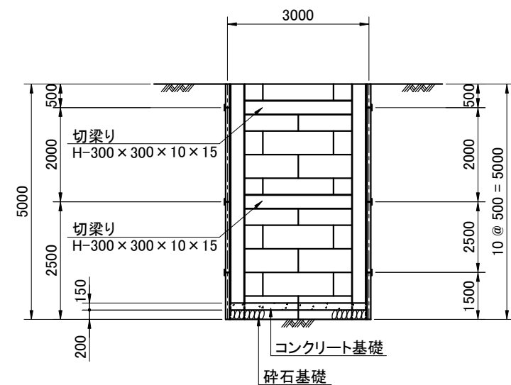
2 - 2 断面図
