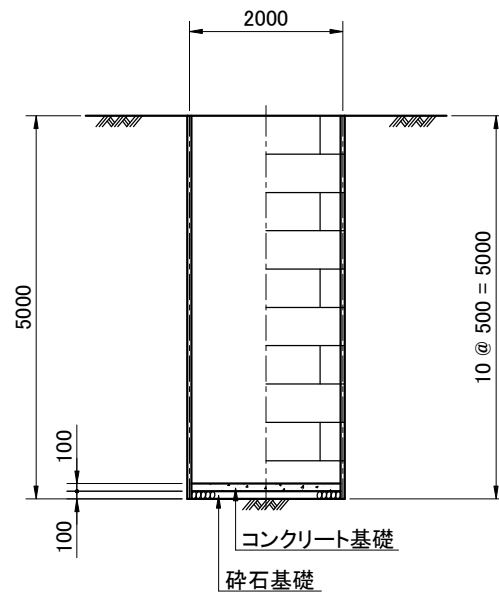
1 - 1 断面図
