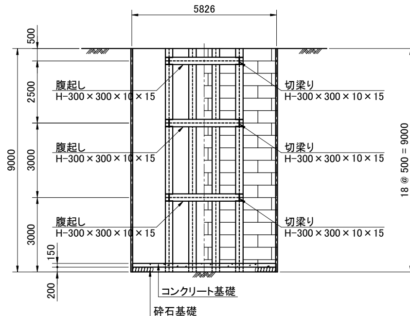
1-1 断面図
