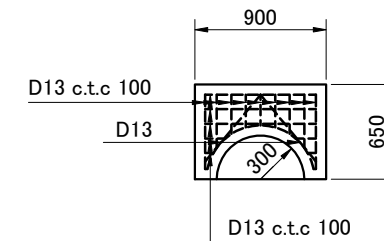
角型 1号
