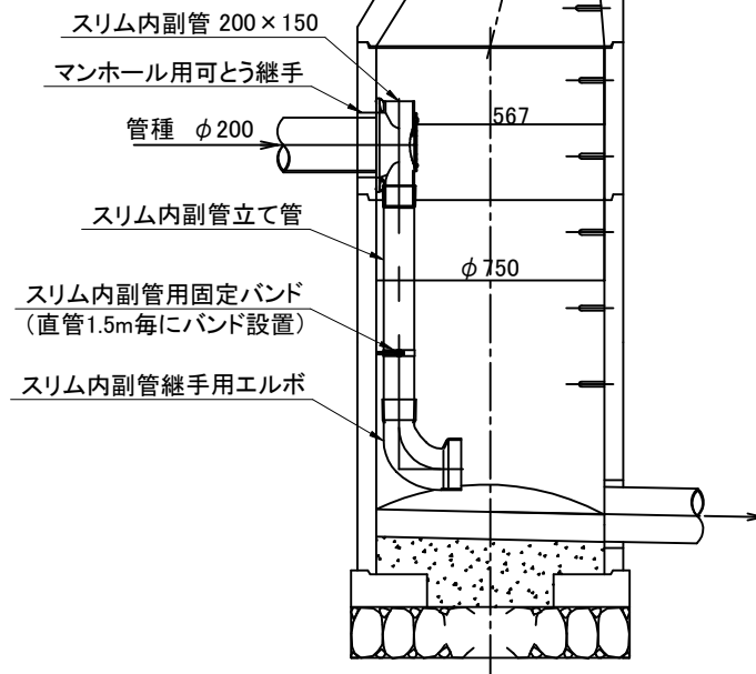
断面図
