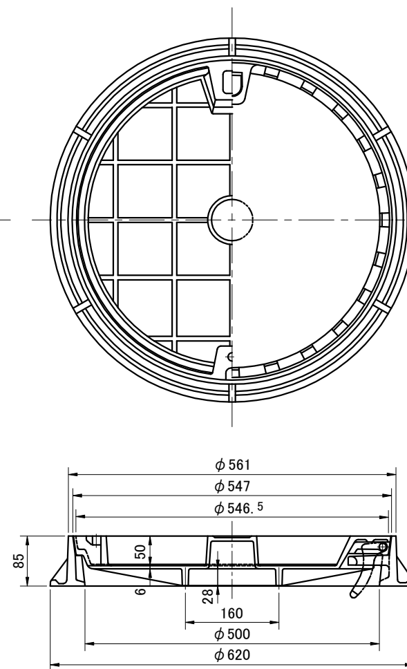
C 型
