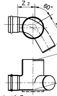
差し口形
