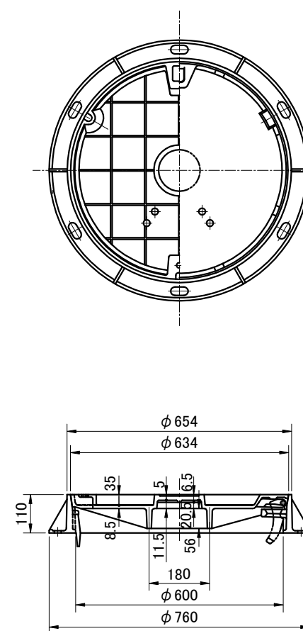
D 型
