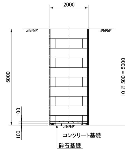
2 - 2 断面図
