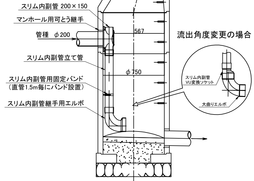
断面図
