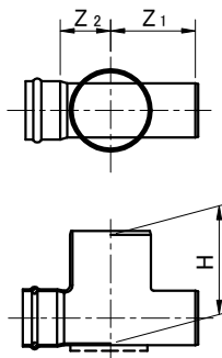
差し口形
