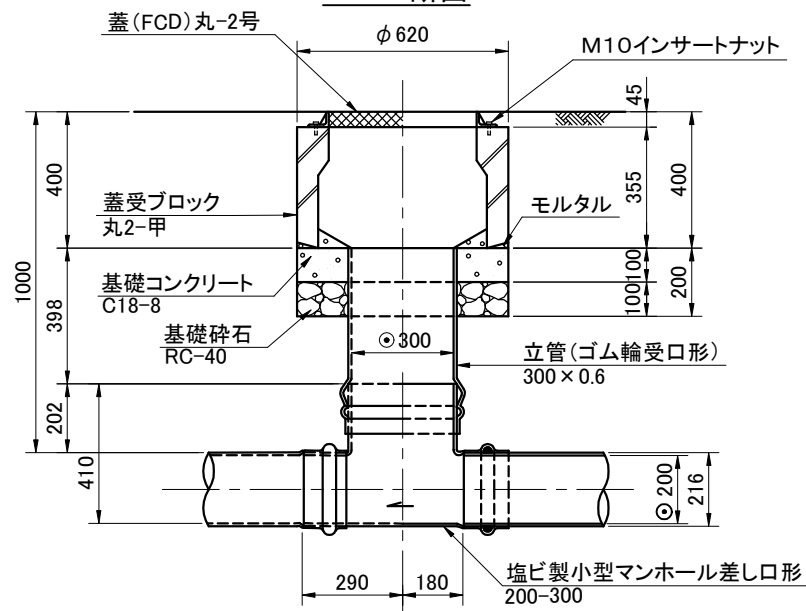
A-A断面
