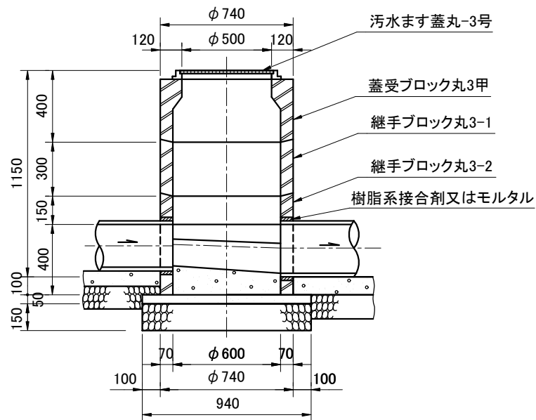
A～A断面図
