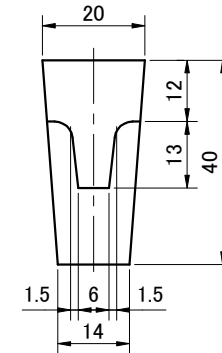
A-A 断面
