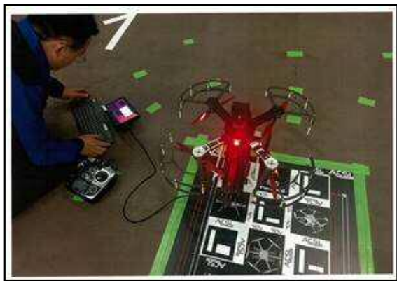
＜写真6＞フライトコントローラーの調整
