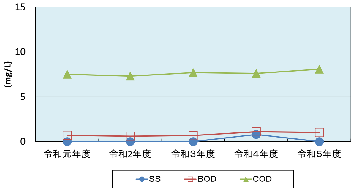
西浄化センター放流水質(平均)の推移
