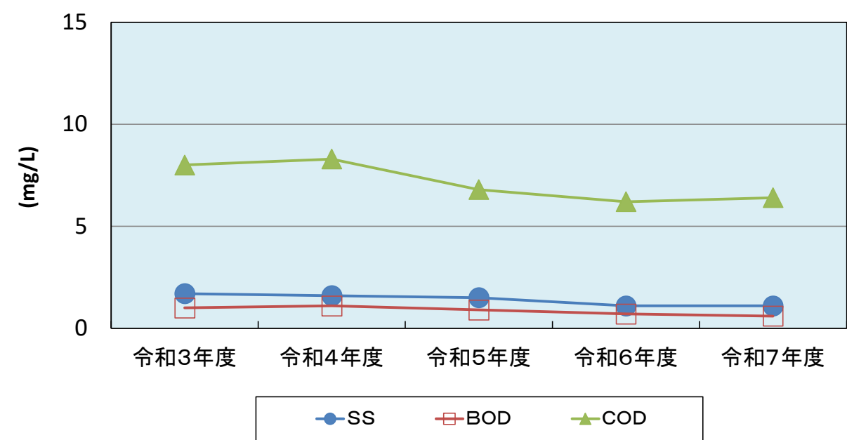
追浜浄化センター放流水質(平均)の推移
